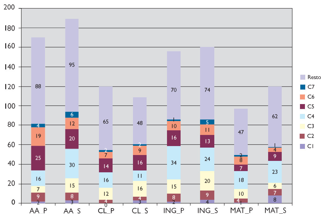
Figura 3. 6 Frecuencia de ítems según la categoría
