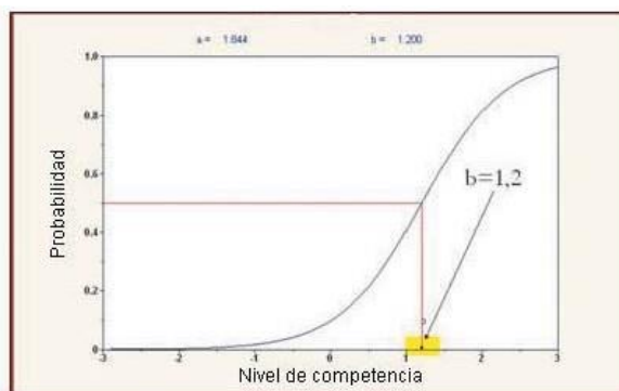
Curva característica del ítem 2
