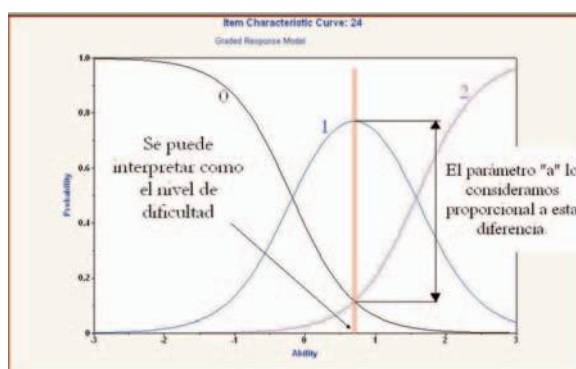
Figura A2. 7 Aproximación al «nivel de discriminación» en ítems politómicos
