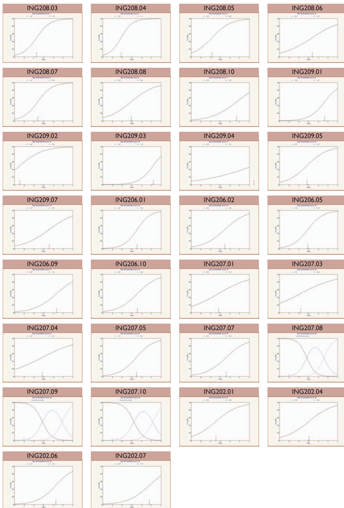
Figura A2. 13 Curvas características de los ítems
