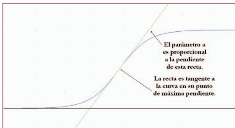
Figura A2. 3 Parámetro a . Índice de discriminación
