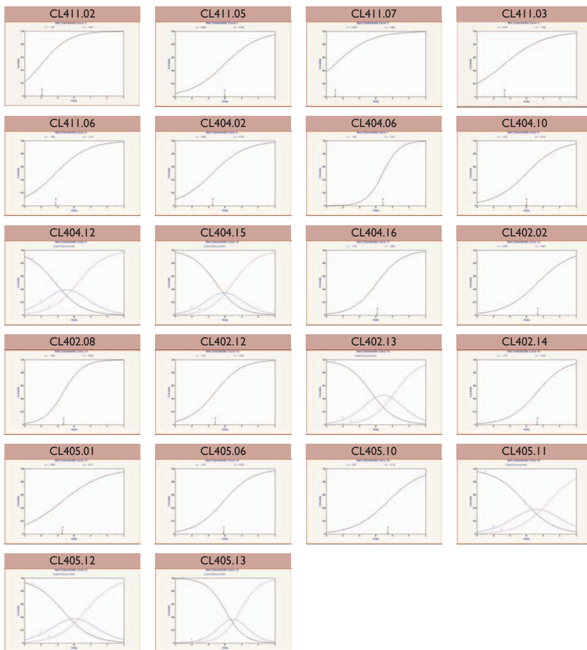
Figura A2. 16 Curvas características del ítem
