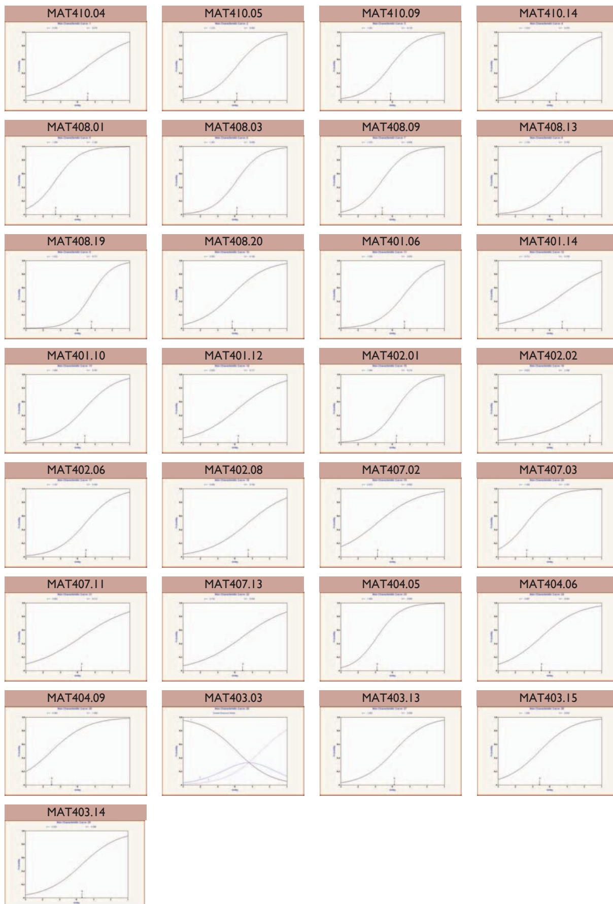
Figura A2. I8 Curvas características del ítem
