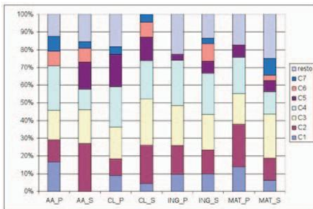
Figura A2. 12 Gráfico de porcentajes en las pruebas definitivas. Categorización de ítems
